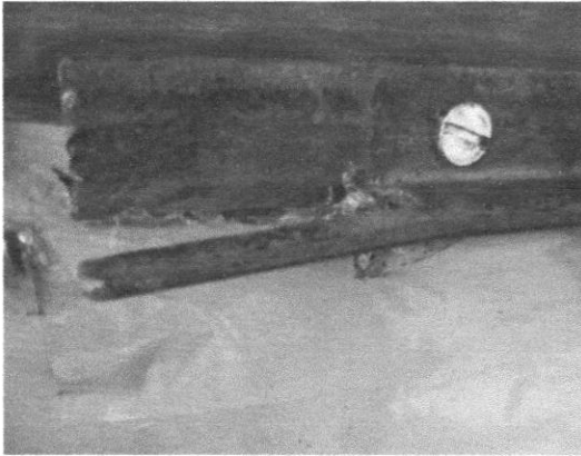
Foto 07: Corrosão no encaixe inferior do Quadro Servo de Deus
